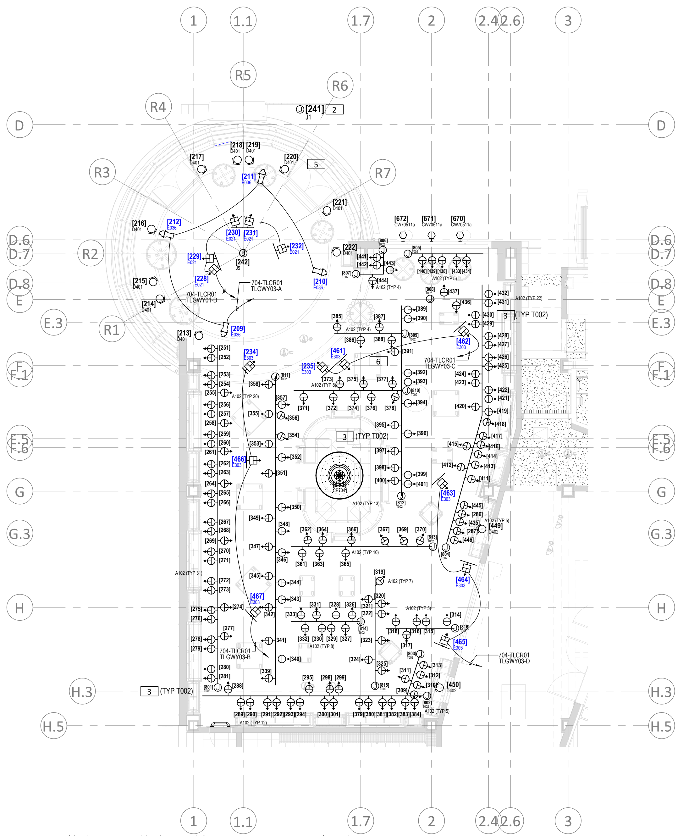
天花板平面图 - 首层f区 - 主题灯光 CEILING PLAN - LEVEL1 AREA f - THEMED LIGHTING
