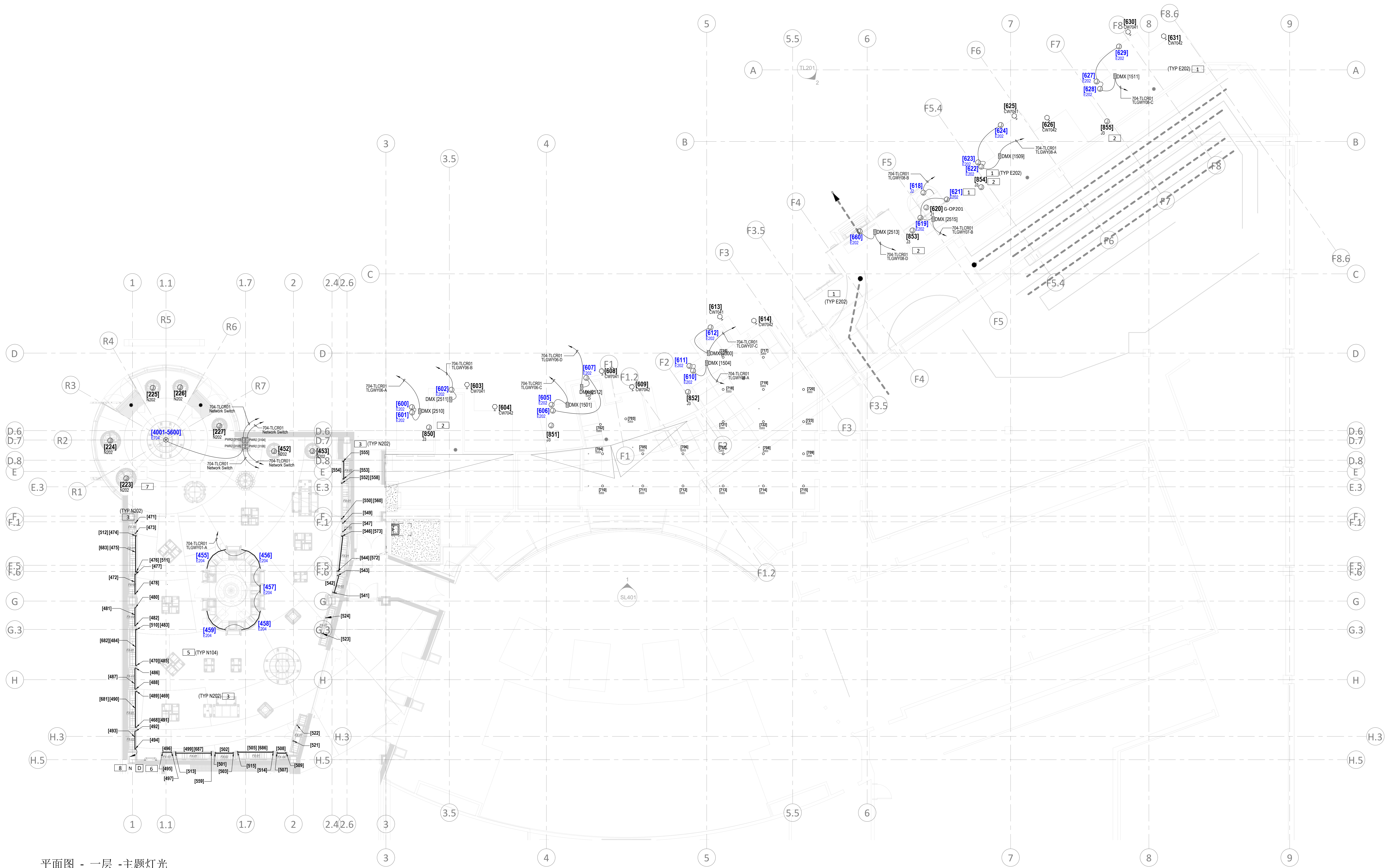
平面图 - 一层 - 主题灯光 Plan View - Level1 - THEMED LIGHTING
